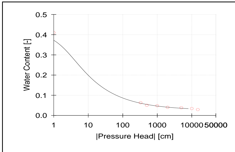
الشكل 1 منحنى وصف رطوبة التربة الوزني
